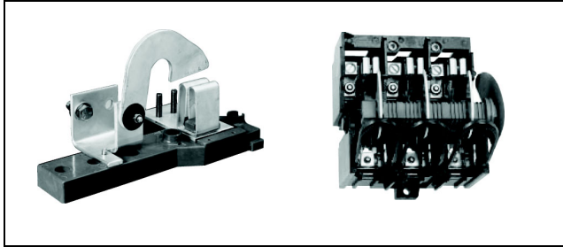
FIG. 3 : Examples of Line Base Assemblies / Ejemplos de ensamblajes de la base de línea / Exemples d'assemblages de la base de ligne
