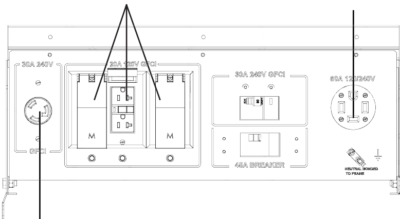
NEMA L6-30R 30A
