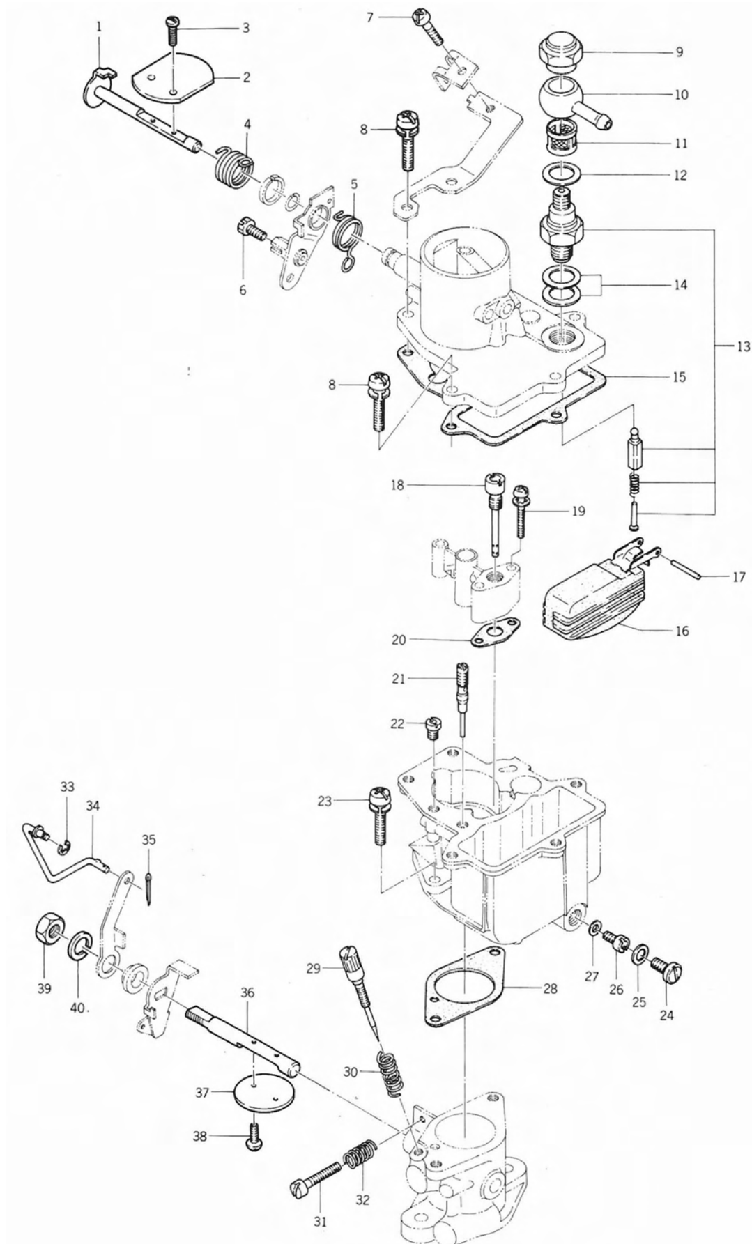
Fig. C-1 CARBURETOR
