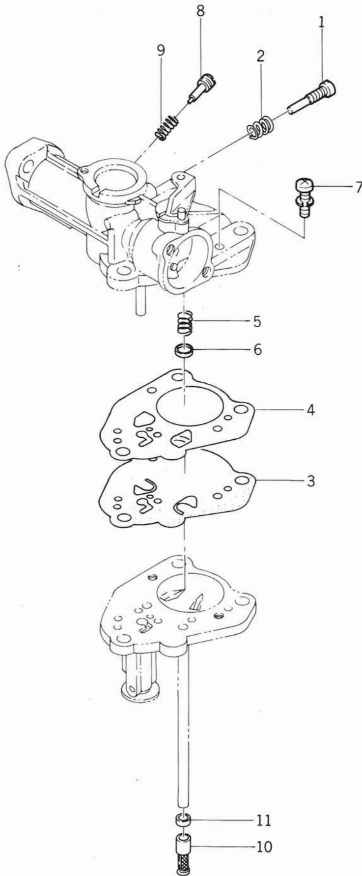
Fig. C-1 CARBURETOR
