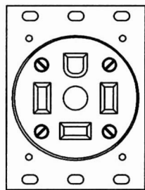
NEMA: 14-60R 125/250V-60A
