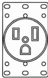
NEMA 6-50R 250V-50A
