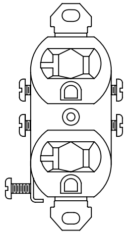
NEMA: 5-20R 125V-20A
