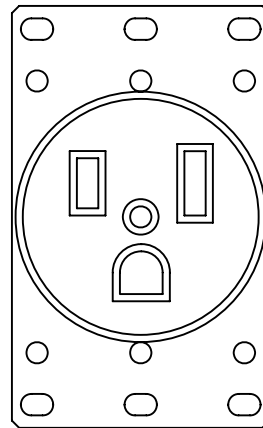
NEMA 6-50R 250V-50A
