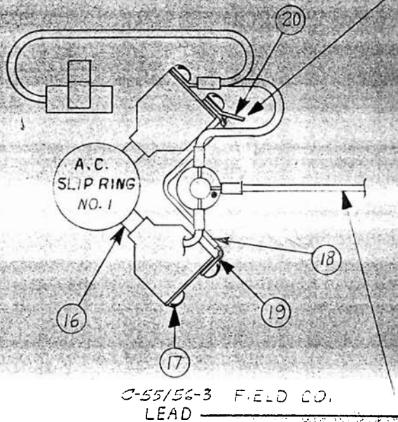
WIRING DIAGRAM 55295
