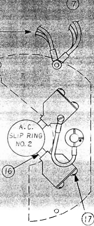
WIRING DIAGRAM 55295
