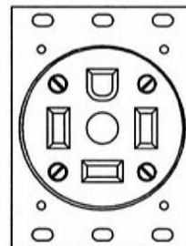
NEMA: 14-60R 125/250V-60A
