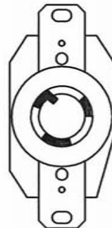
NEMA: L5-20R 125V-20A
