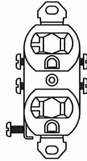
NEMA: 5-20R 125V-20A
