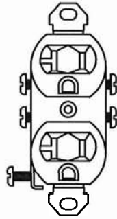
NEMA: 5-20R 125V-20A
